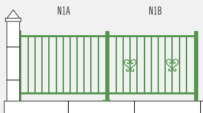
SIMPLES 2 TRAVERSES BARREAUX Ø20
